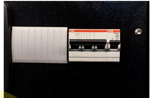
Электрическая часть ДГУ производства ABB
